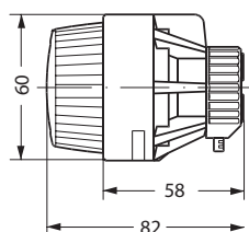
RTR 7094 (модель с защитным кожухом)
