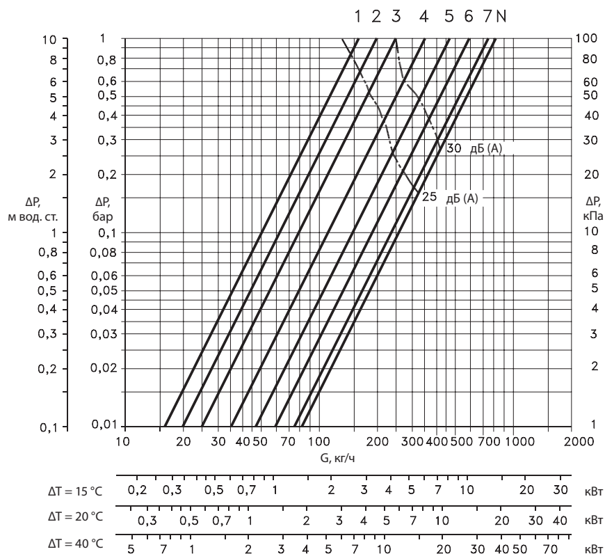
Диаграмма для определения предварительной настройки клапана RTR-N 20 UK
