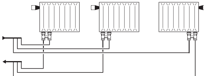
Двухтрубная горизонтальная система отопления
