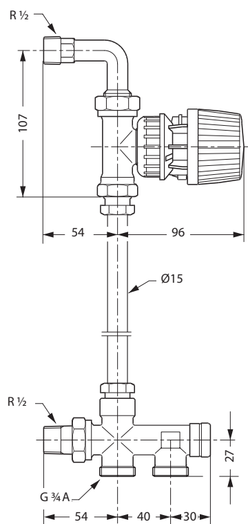
RTR-K с нижним подключением, G 3/4 A, с термостатическим элементом RA2994
