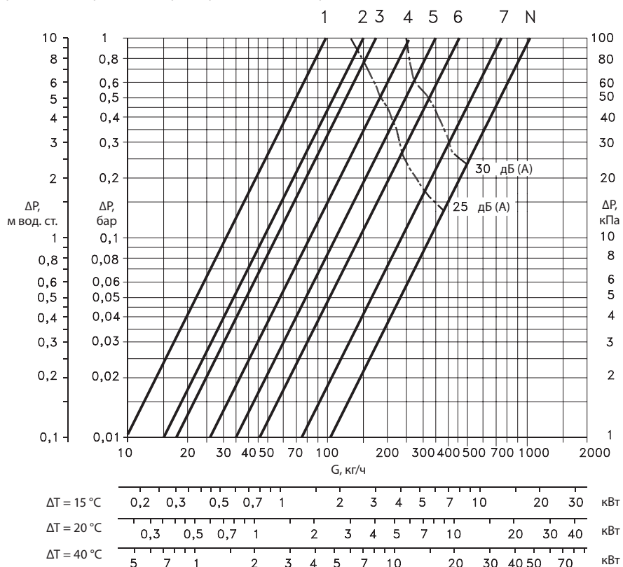
Диаграмма для определения предварительной настройки клапана RTR-N 20/25
