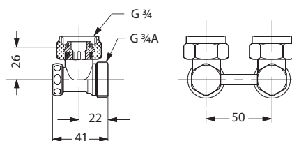
RLV-KS угловой с присоединением к отопительному прибору G ¾
