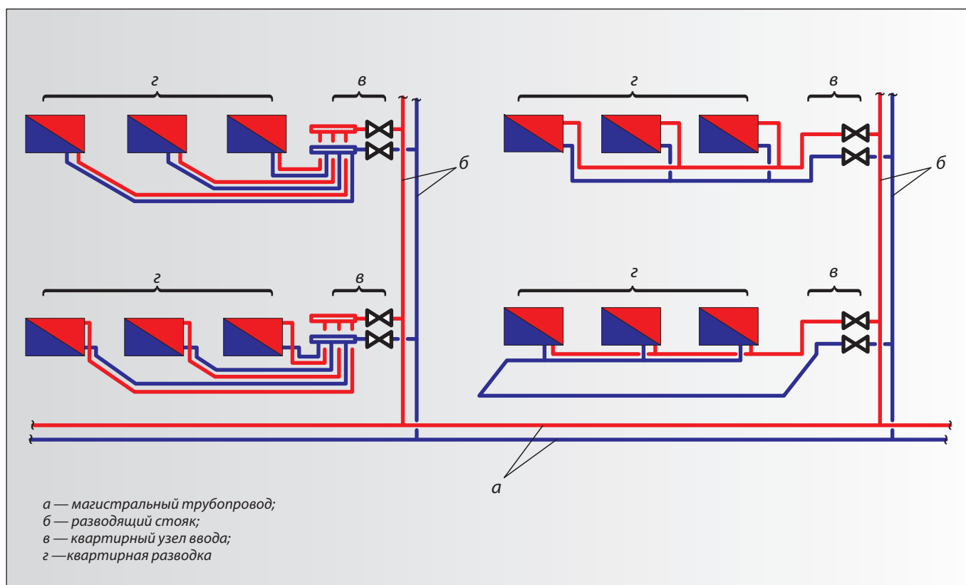
Рис. 34. Принципиальная схема поквартирной системы отопления многоэтажного здания.
