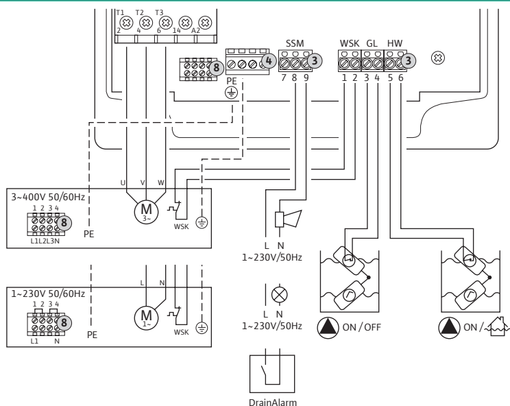
Прибор управления MS-L-1 без главного выключателя, без кабеля и штекера
