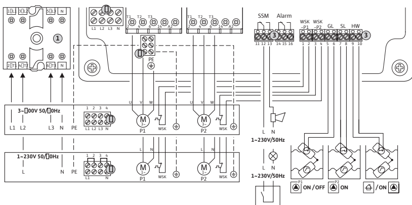
Прибор управления MS-L-2 с главным выключателем
