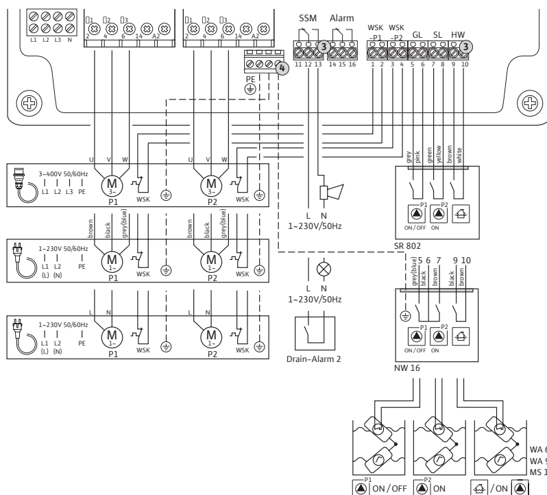
Прибор управления MS-L-2 без главного выключателя, с кабелем и штекером
