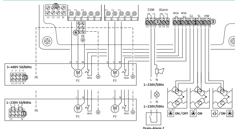
Прибор управления MS-L-2 без главного выключателя, без кабеля и штекера
